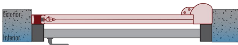
CORTE HORIZONTAL
