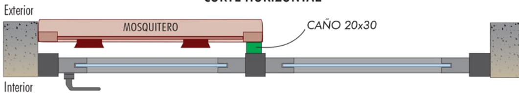
CORTE HORIZONTAL
